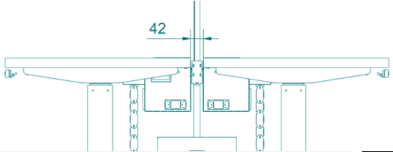
Distancia central entre superficies para pantalla Acústica tapizada
