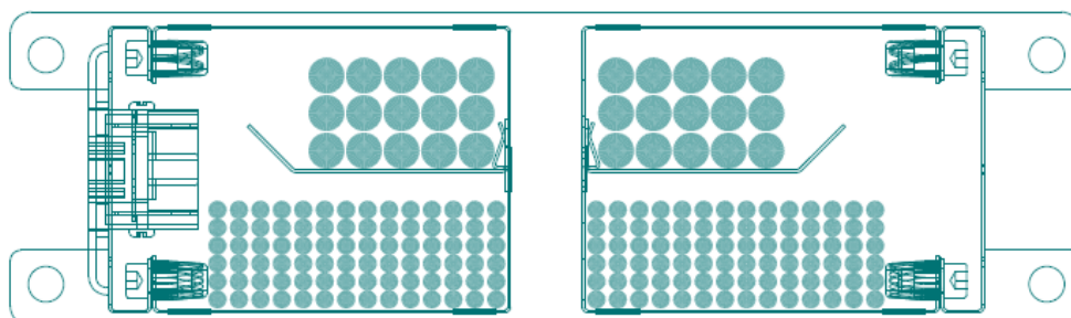
84 cables de poder No. 10 / 12 (diámetro 5mm)
