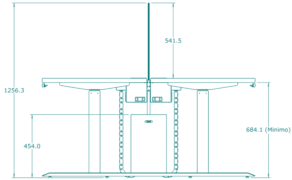
Dimensiones en milímetros (mm)
