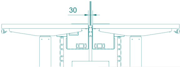
Distancia central entre superficies para pantallas vidrio laminado, formica y melamina
