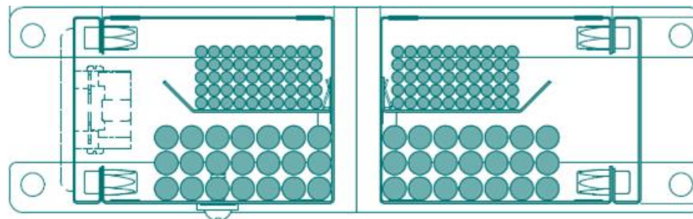
21 cables UTP categoría 6A / 7 (diámetro 10mm)
